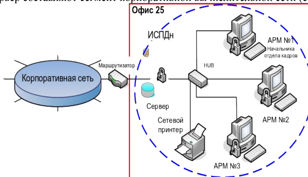
Схема ИСПД «Кадры» ЗАО «Солнышко»
