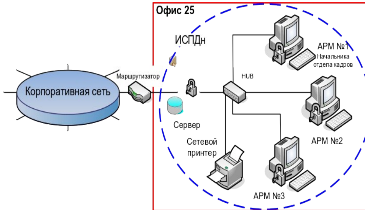
Рисунок 1 – Схема ИСПДн «Кадры» ЗАО «Солнышко»
